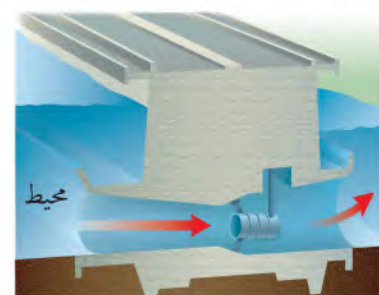
أ خلال المد تدير حركة الماء التوربين المرتبط مع المولد الكهربائي، وعند اكتمال المد تغلق البوابة لتحبس الماء خلف السد.
