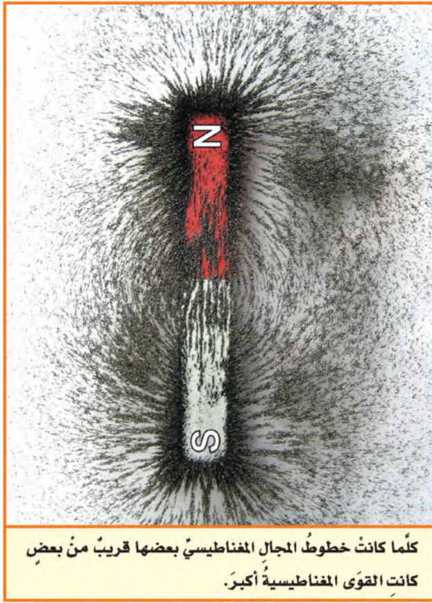
يشبه المجال المغناطيسي للأرض المجال المغناطيسي لقضيب مغناطيسي.
